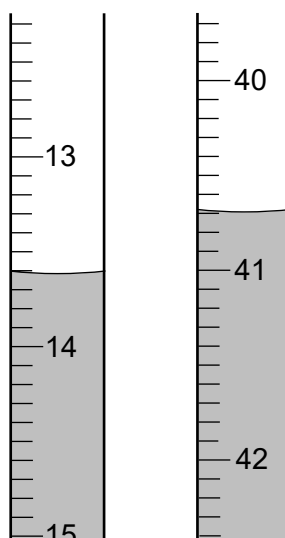
2nd titration
